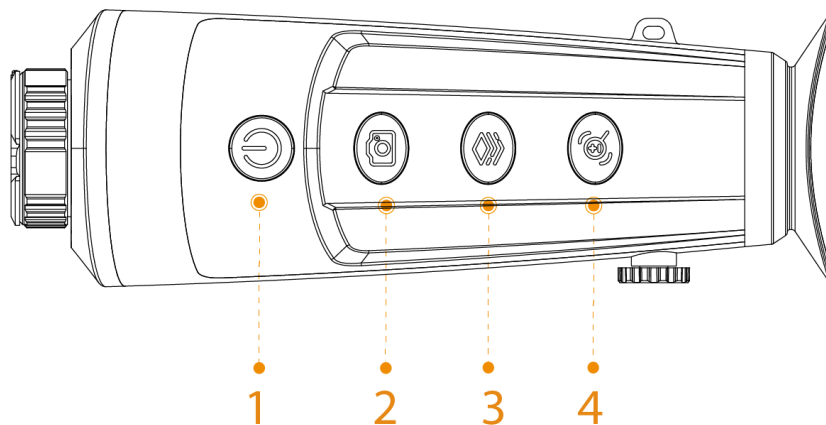
Рисунок 2-2 Описание кнопок (50 мм)
