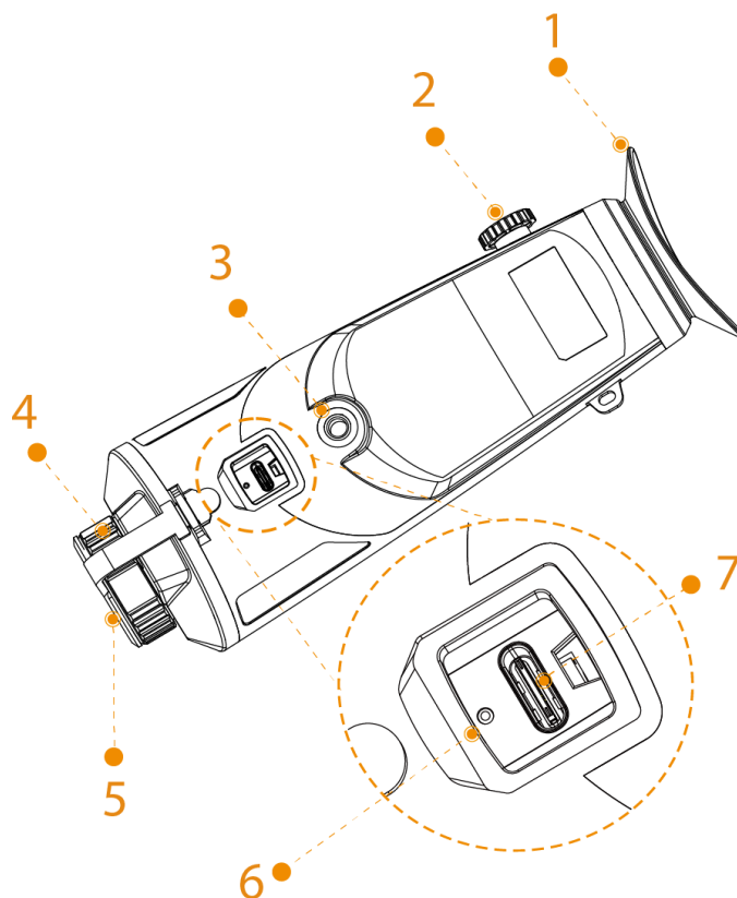
Рисунок 2-4 Описание порта (50 мм)
